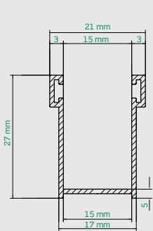
Cod. guida 919 (da sostituzione) 28x17x28 mm
