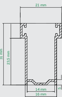
Cod. guida 36764 (da sostituzione) 31x16x31 mm
